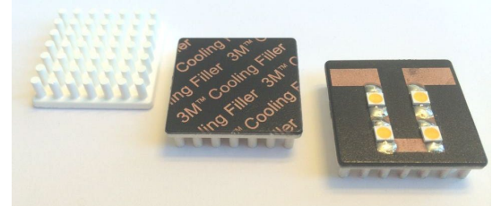
LEDデバイスのヒートシンク (PETベース、1.5W/mK品)
